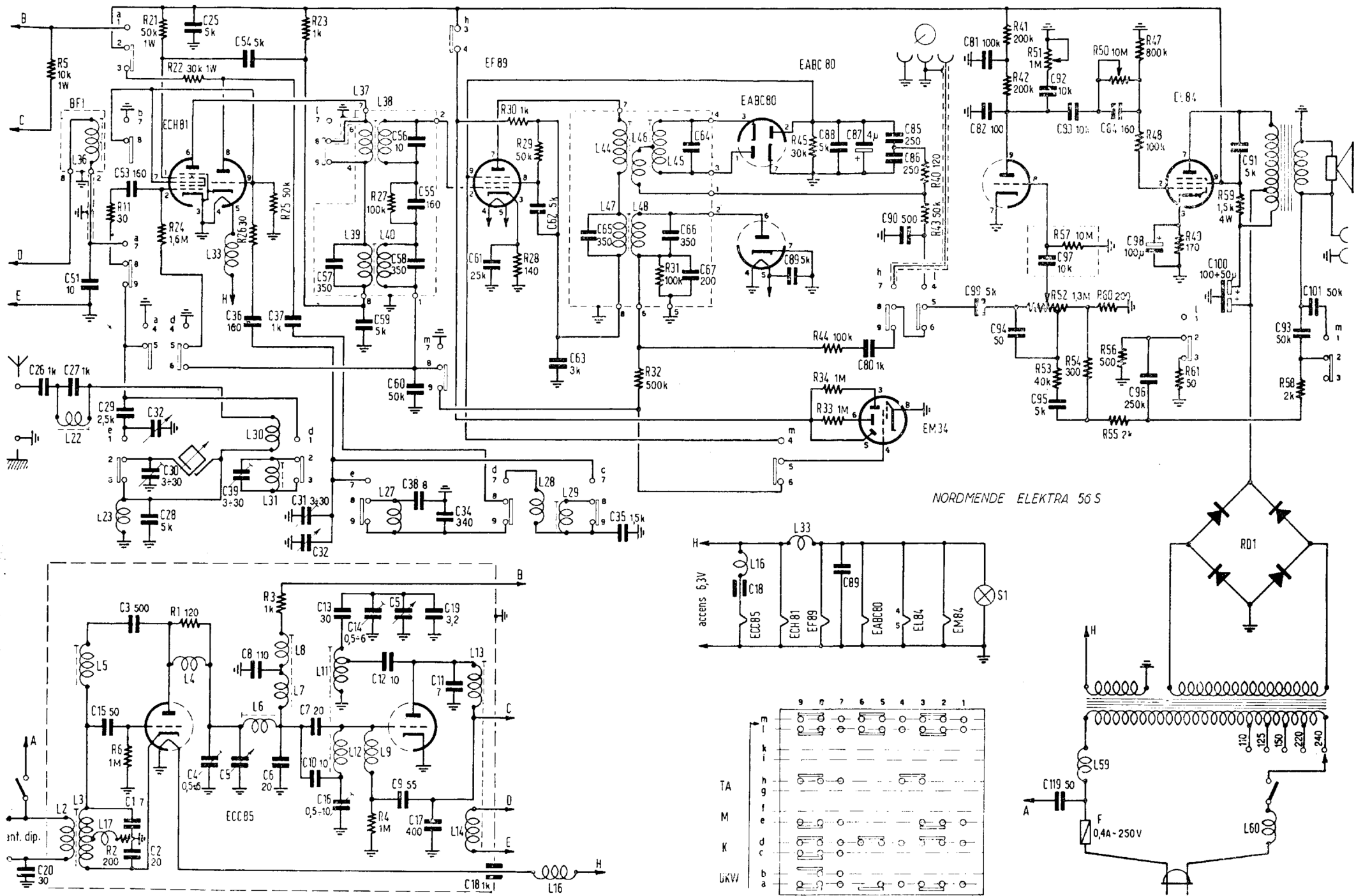
SCHEMA ELETTRICO DEL RADIORICEVITORE AM-FM NORDMENDE ELEKTRA 56 S
